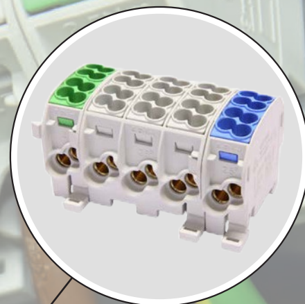
Инновационный механизм фиксации на DIN рейке
