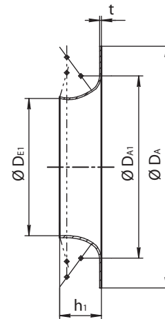
Конфузор типа ED 10
