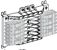
4 ways (3P)
