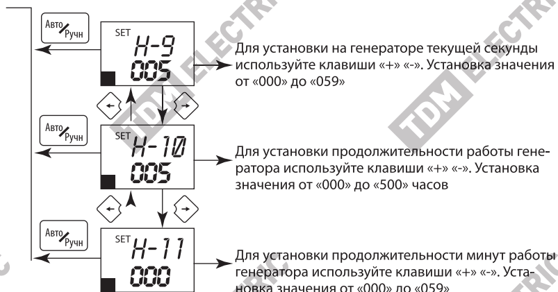
Рисунок 7. Режимы работы АВР-ПНД, установка режимов работы генератора
