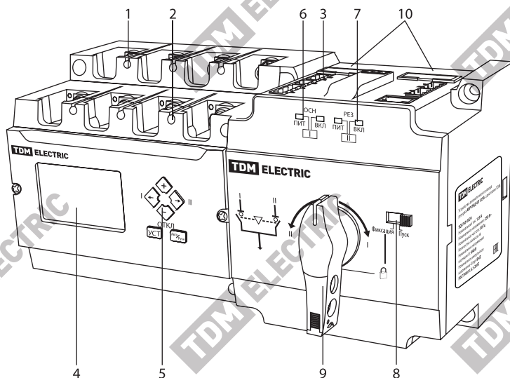
Рисунок 9. Внешний вид АВР-ПНД
