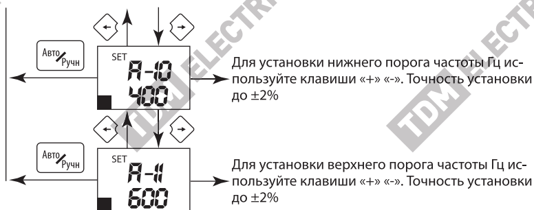
Рисунок 5. Режимы работы АВР-ПНД, основное меню
