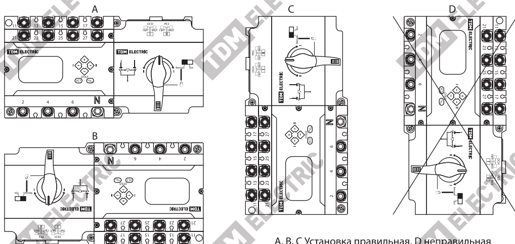
Рисунок 2. Установка переключателя
