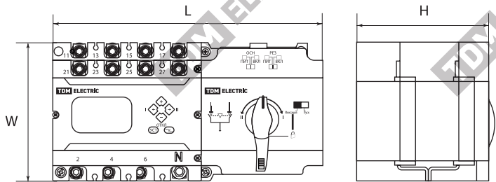
Рисунок 10. Габаритные размеры АВР-ПНД
