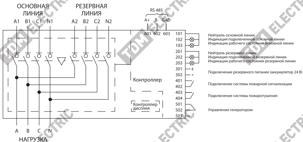
Рисунок 1. Схема подключения АВР-ПНД
