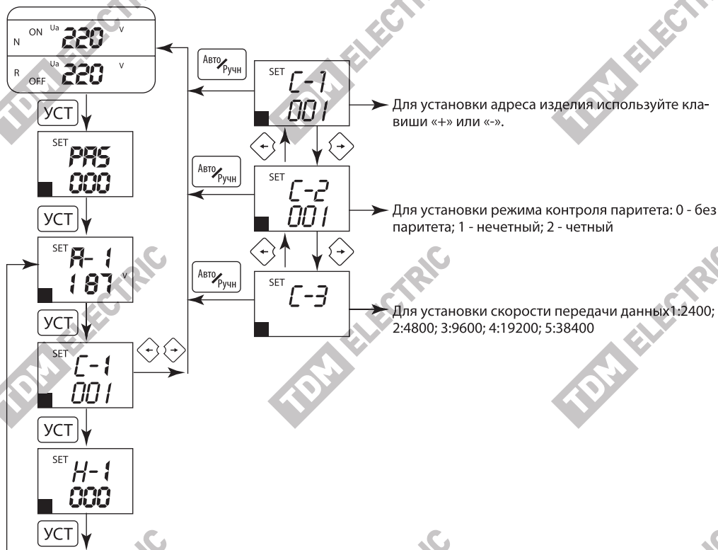
Рисунок 6. Режимы работы АВР-ПНД, установка RS485 Modbus
