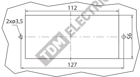
Рисунок 11. Окно под выносную панель
