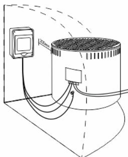
Рисунок 4 – Схема подключений
