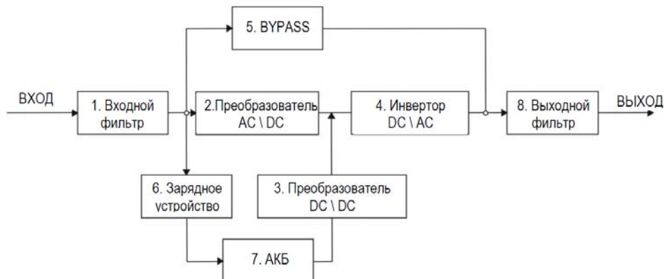
Рисунок 4 - функциональная схема изделия
