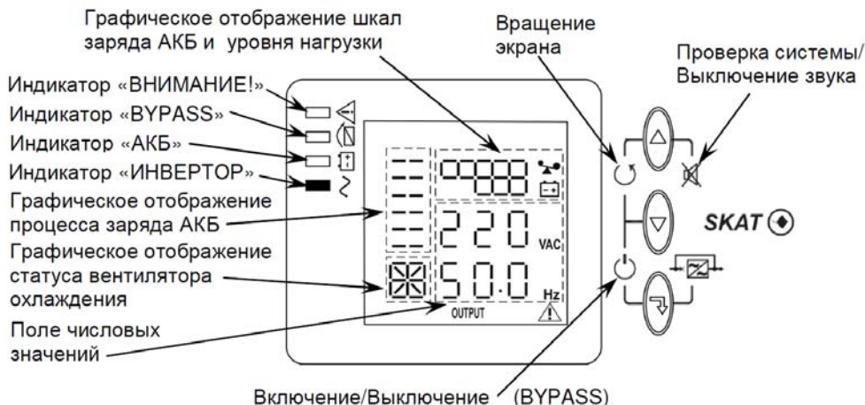
Рисунок 1 - Передняя панель изделия при монтаже в горизонтальном положении (на ЖК-дисплее отображены выходные параметры изделия (экран OUTPUT))
