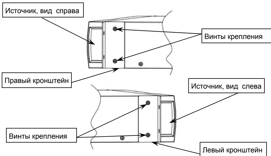
Рисунок 7 — установка кронштейнов на корпус изделия
