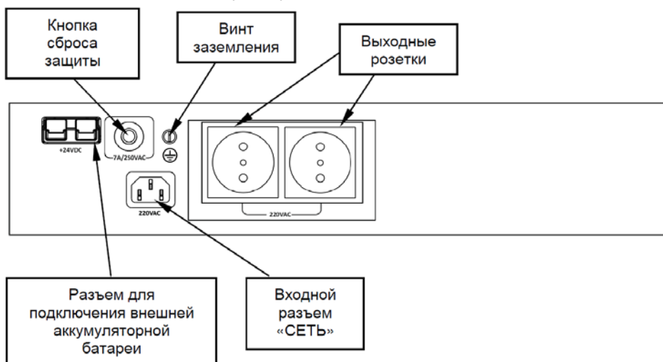
Рисунок 3 - задняя панель изделия при монтаже в горизонтальном положении
