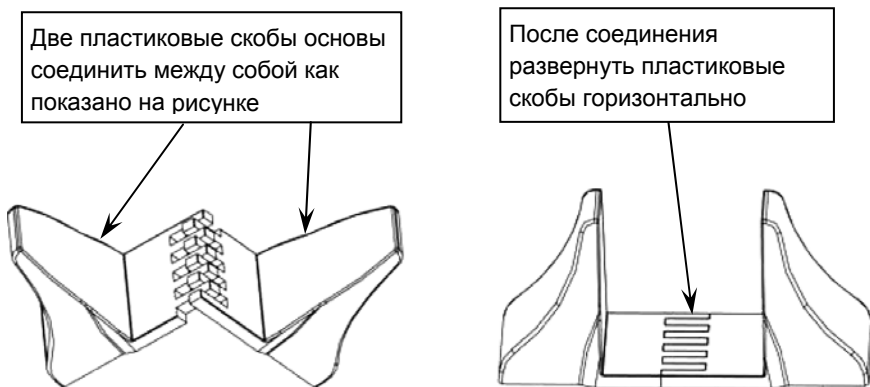
Рисунок 5 - сборка пластиковых основ для вертикальной установки изделия
