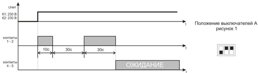
Рисунок 6 – Алгоритм работы Реле управления (предпусковая сигнализация)
