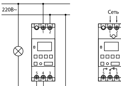
Рисунок 7. Электрическая схема подключения таймера ТЭ15
