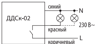
Рисунок 9. Схема подключения датчиков движения ДДСк-02
