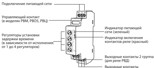
Рисунок 3. Лицевая панель реле
